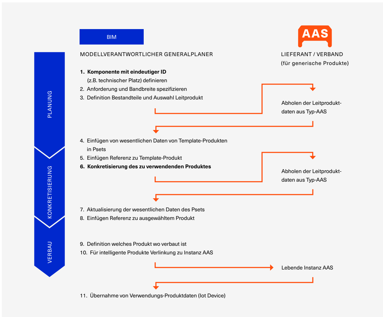
Abbildung 8: Überblick über den Integrationsprozess der AAS-Daten in den BIM-Prozess (syn2tec)
