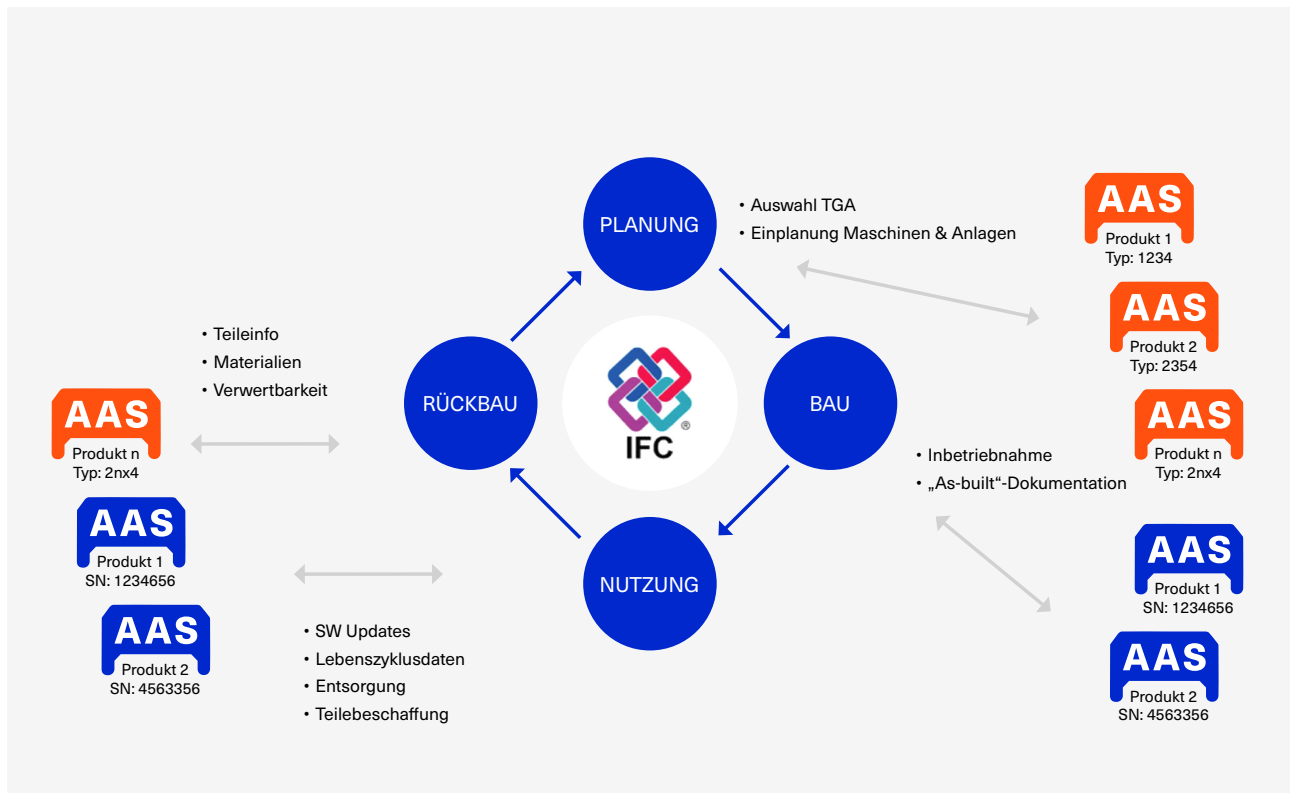
Abbildung 5: Interaktion BIM mit AAS über Lebenszyklus des Gebäudes (syn2tec)
